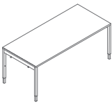
BOY05R 1800 / 800 / 640-860 50.35 kg
